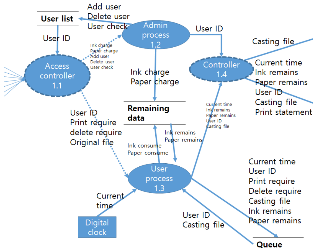
3.2.2.1 DFD
